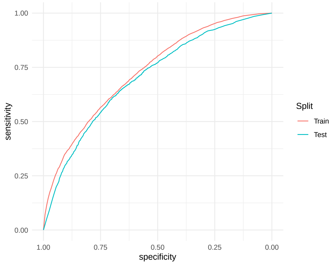
ROC – Train (AUC=0.732) vs. Test (AUC=0.705)
