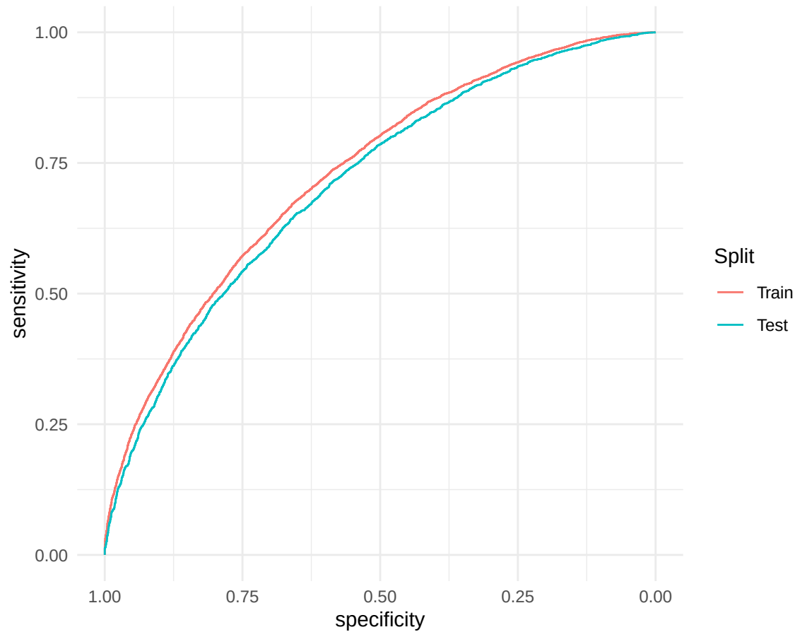
ROC – Train (AUC=0.730) vs. Test (AUC=0.712)
