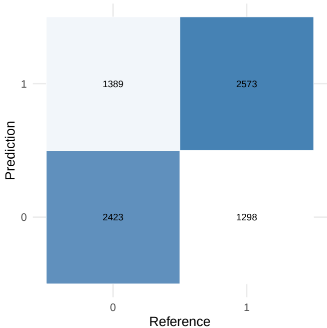
Confusion Matrix (Beispiel)
