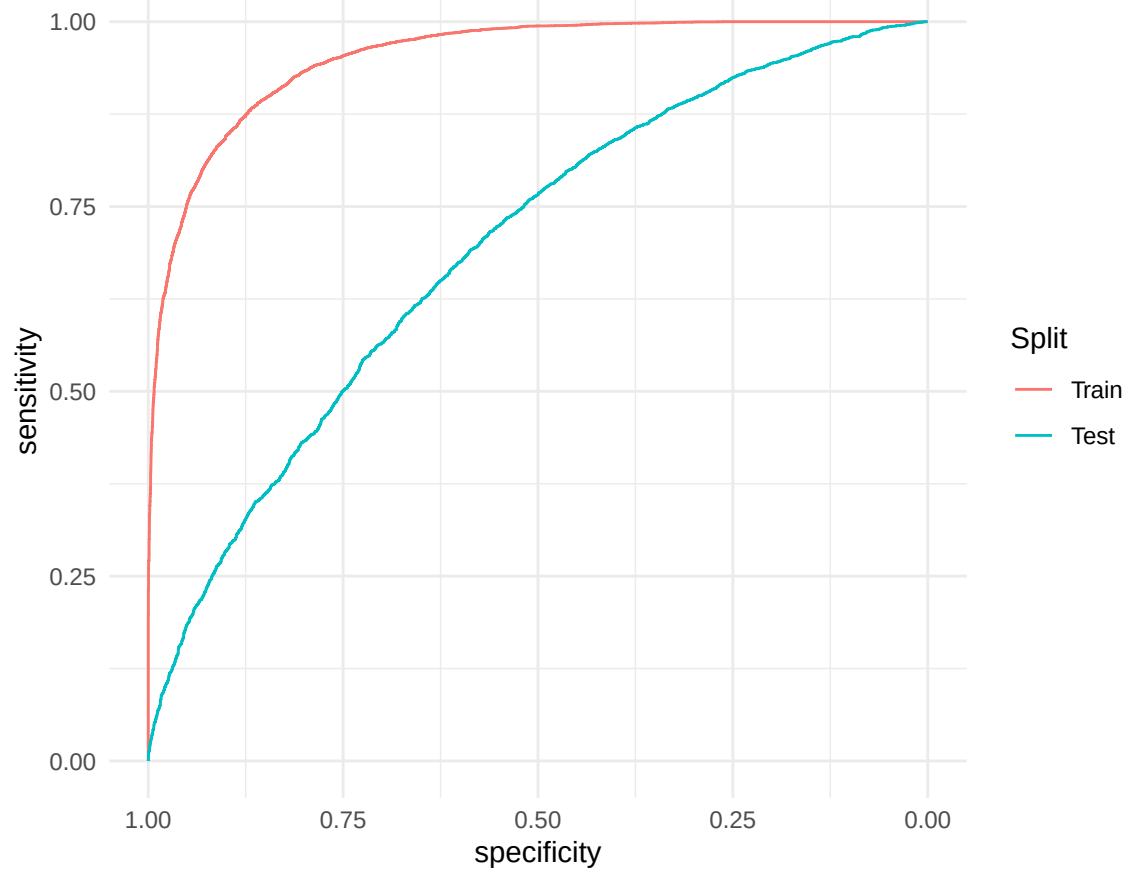
ROC – Train (AUC = 0.952) vs. Test (AUC = 0.692)
