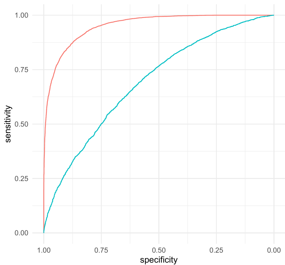
ROC – Train (AUC = 0.952) vs. Test (AUC = 0.692)
