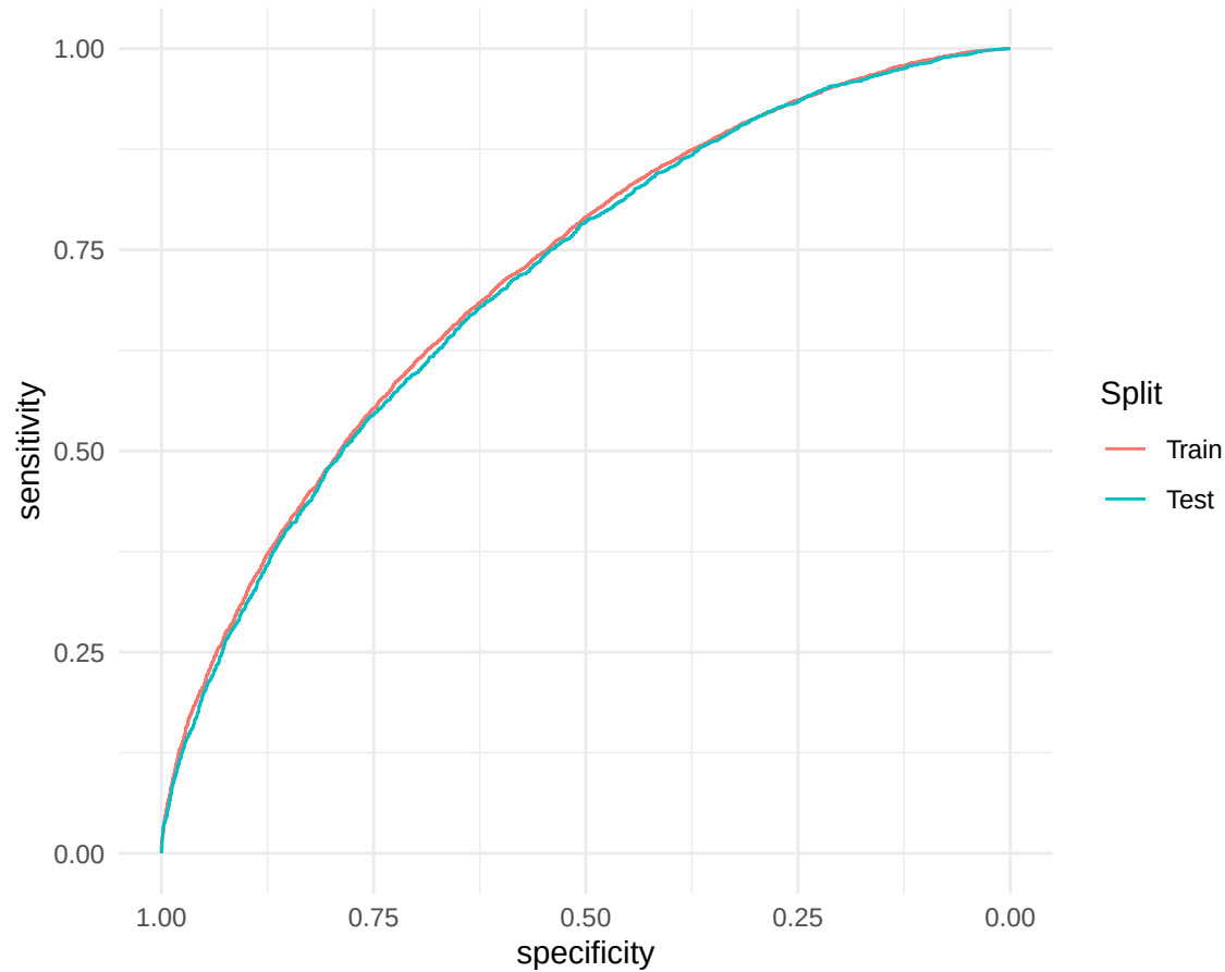
ROC — Train (AUC=0.718) vs. Test (AUC=0.712)
