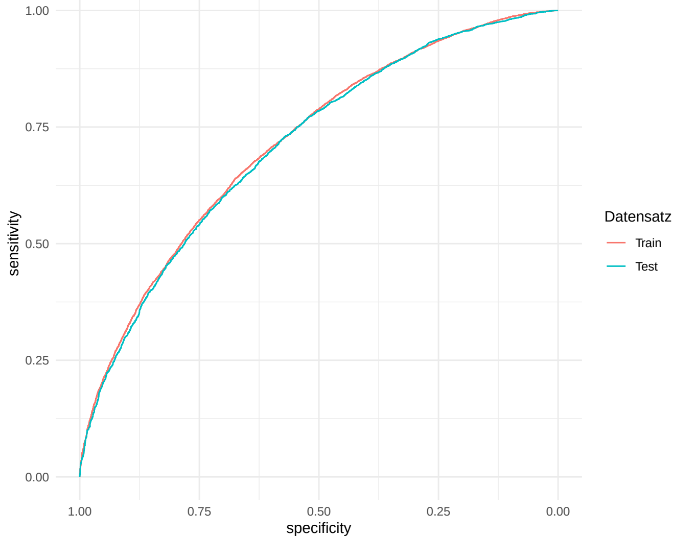
Finale ROC-Kurven — Train (AUC=0.717) vs. Test (AUC=0.712)
