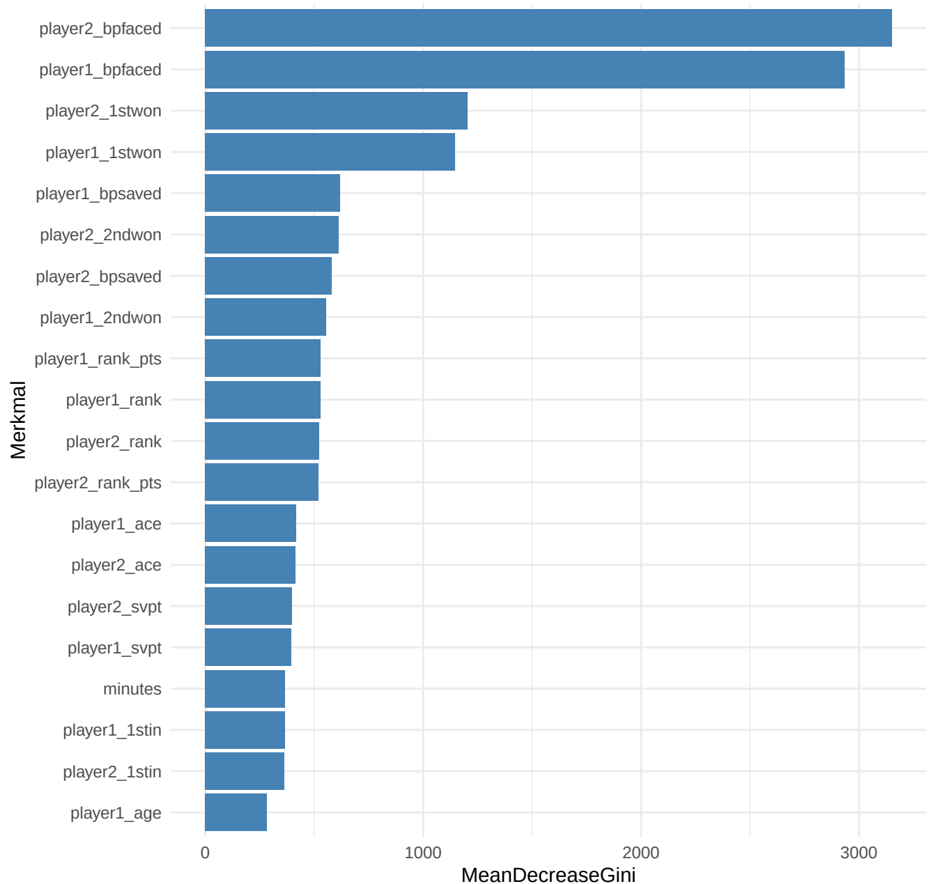
Top 20 wichtigste Merkmale (Random Forest)
