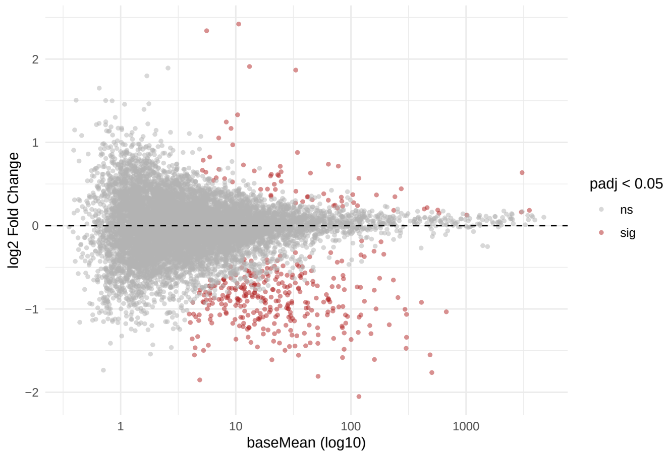
MA plot: CBD vs DMSO
