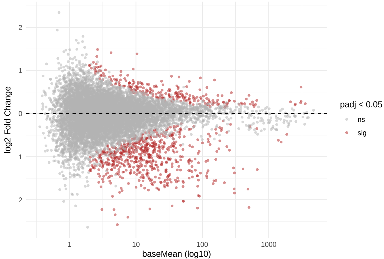
MA plot: THC vs DMSO
