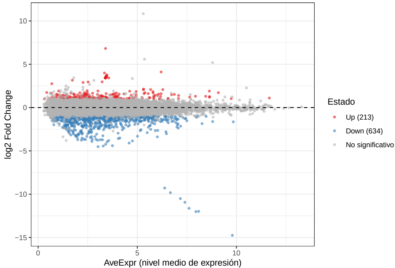
MA plot – Eto_vs_Mock
