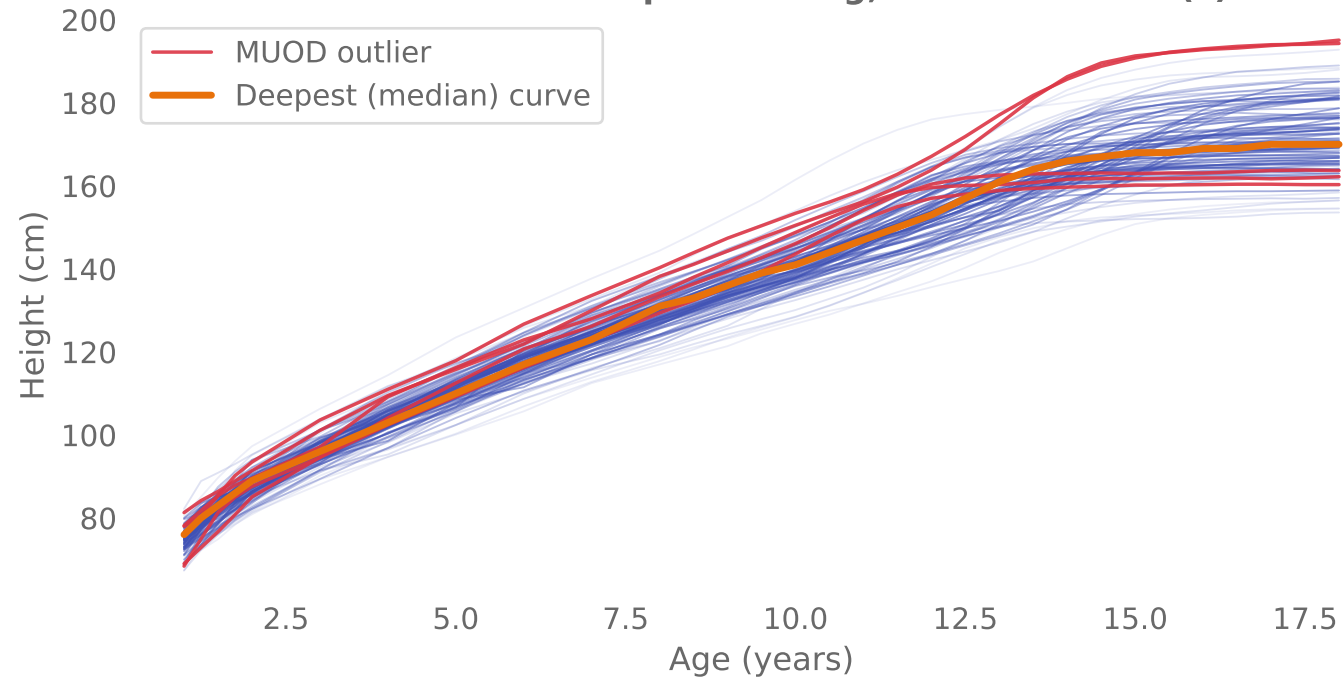
Fraiman--Muniz depth shading; 5 MUOD outlier(s)
