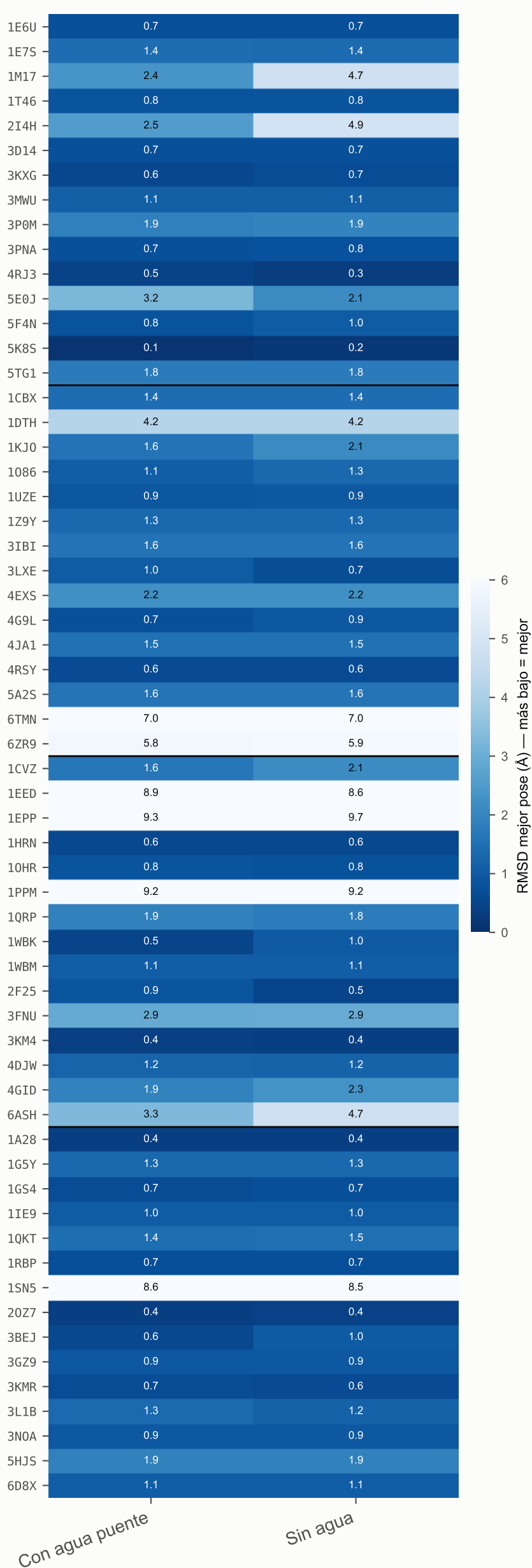
Figura — RMSD (mejor de 9 poses) por caso y política 60 casos, agrupados por estrato de riesgo
