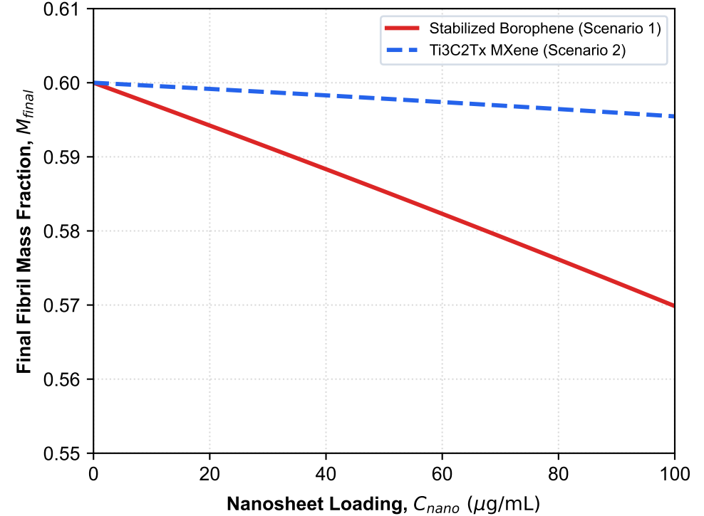
(d) Fibrillation Reduction M_{final}
