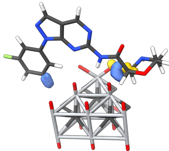
(b) Glioblastoma / Ti 3 C 2 O 2 MXene
