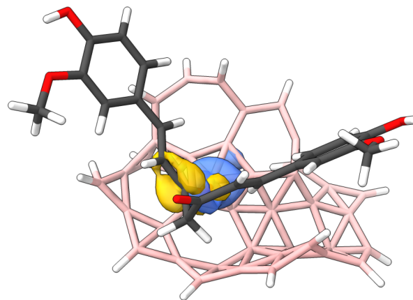
(d) Alzheimer's Tau / \beta 12 borophene
