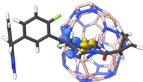
(c) TNBC / B36N36 nanocage
