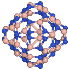
a B 36 N 36 (GP(1,1), 108 B–N)
