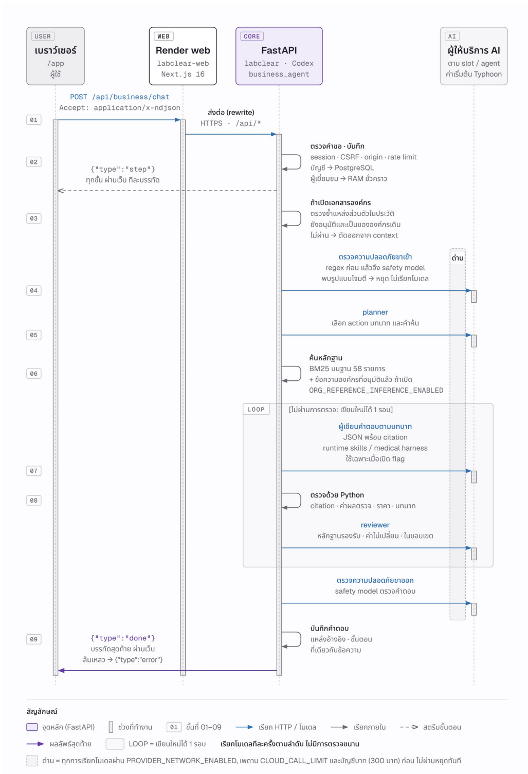
ภาพที่ 3 การไหลของข้อมูลของ 1 ข้อความในแชต รุ่น 4.0.0-rc1
