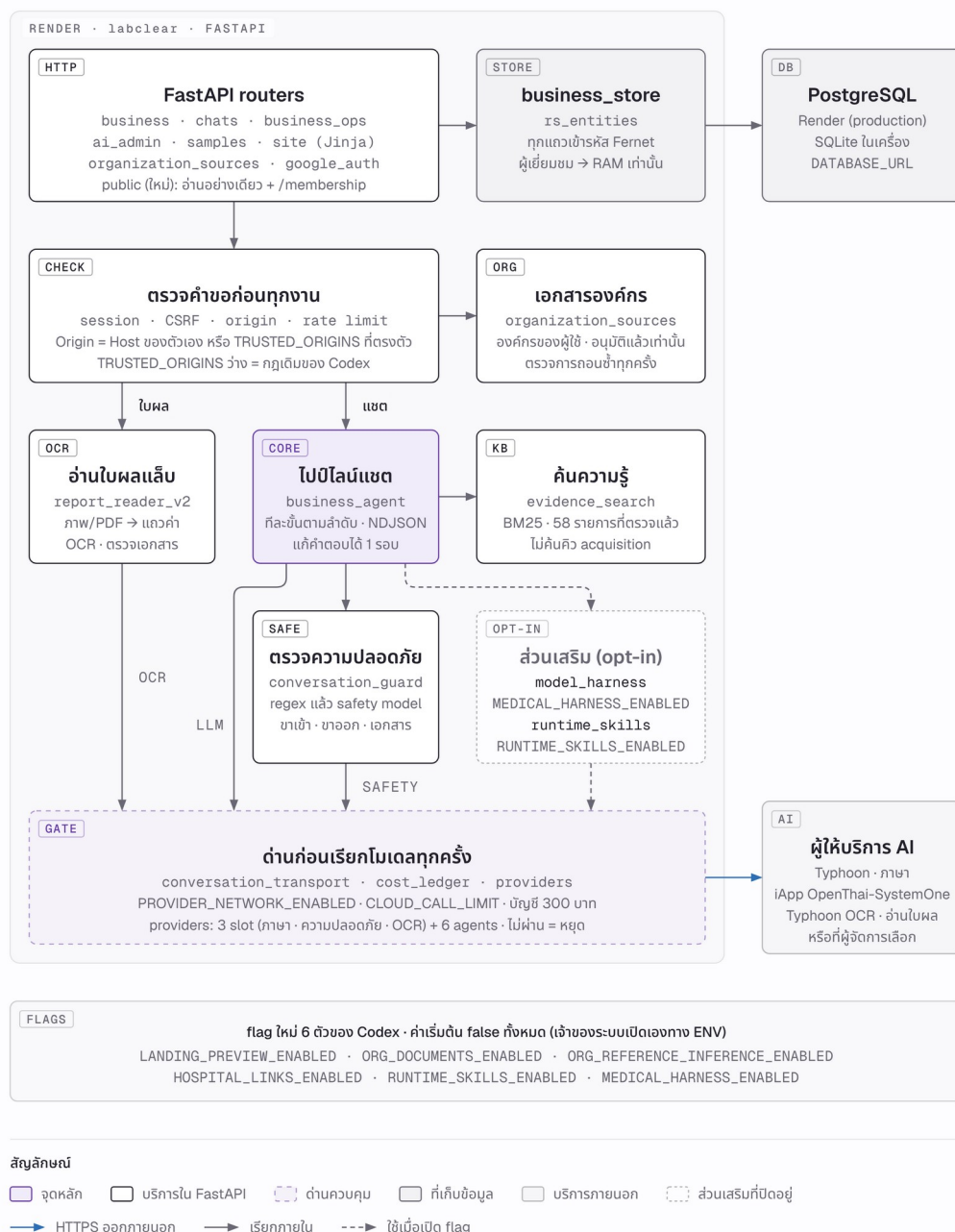
ภาพที่ 2 องค์ประกอบภายใน FastAPI ของ LabClear รุ่น 4.0.0-rc1
