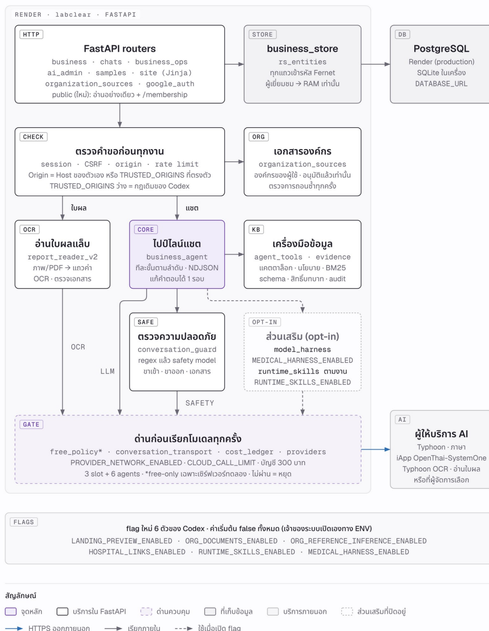
ภาพที่ 2 องค์ประกอบภายใน FastAPI ของ LabClear รุ่น 4.0.0-rc2
