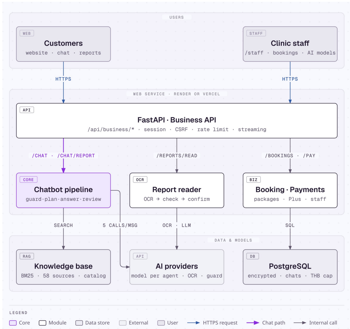
ภาพที่ 1 สถาปัตยกรรมของ LabClear
