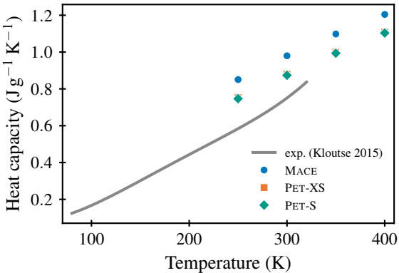
MOF-177
