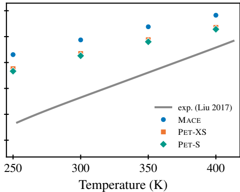
MIL-101
