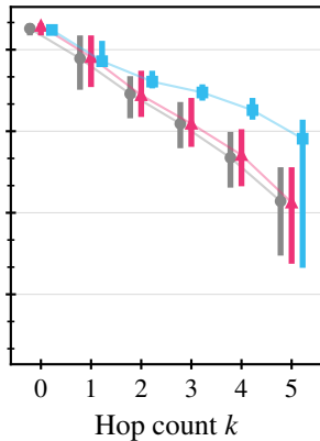
PET-XS
