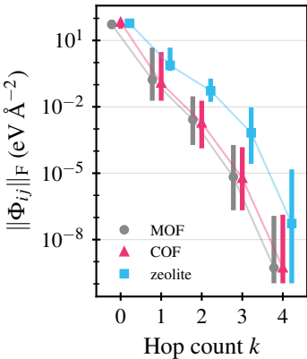
MACE
