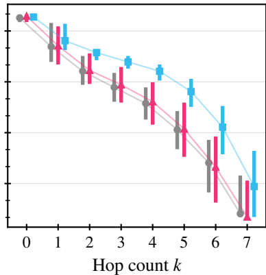
PET-S
