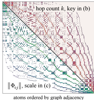
(d) Hessian
