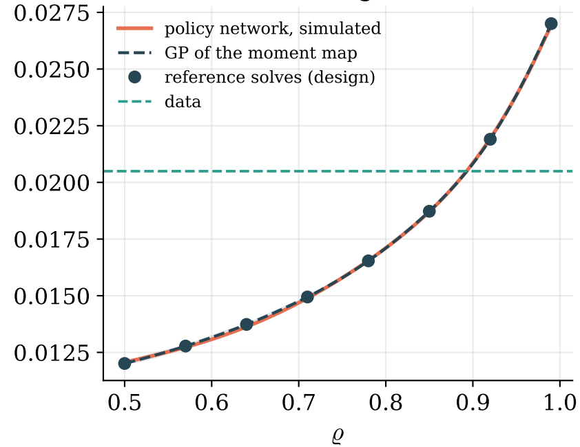
Std(dlog C)
