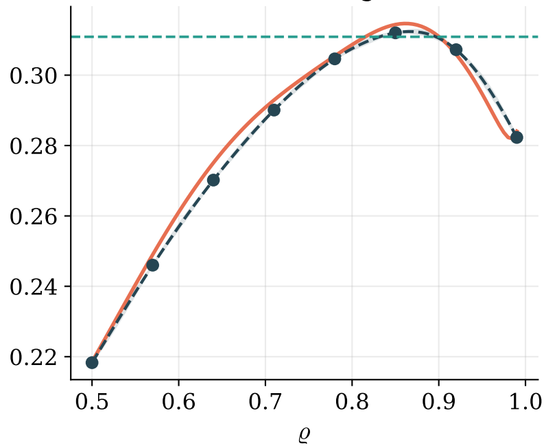
Autocorr(dlog C)
