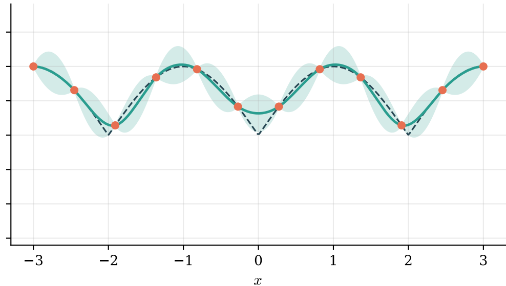
Matérn 3/2, log ML -8.3
