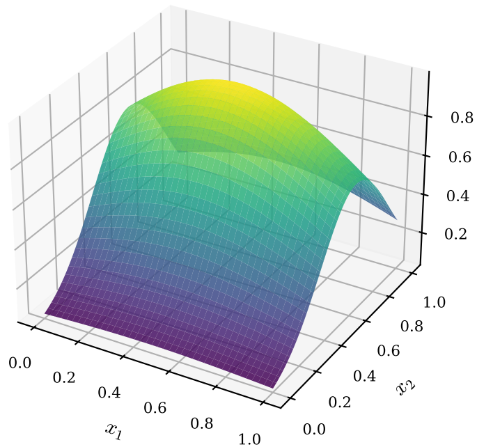
true f(\mathbf{x})
