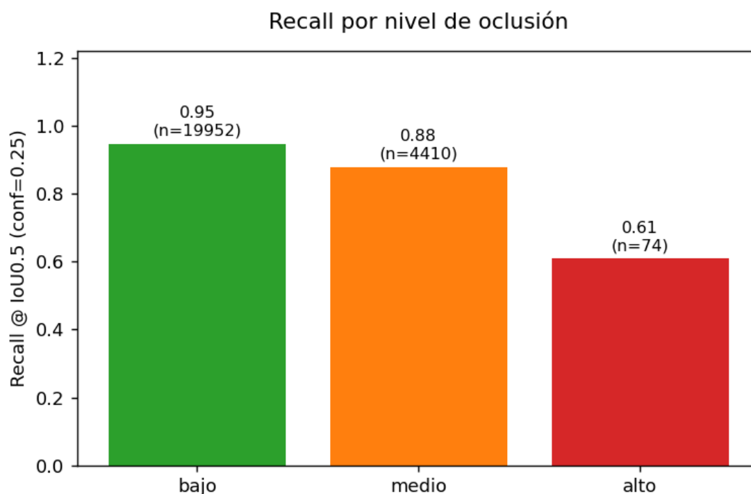
Figura 5. Recall por nivel de oclusión estimado.
