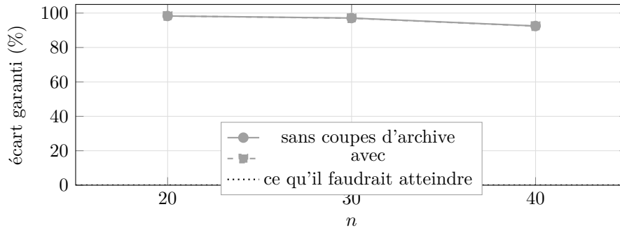
FIGURE 15 – Version antérieure , configuration [V_0 \text{ So } D_0] , budget en temps. Les deux courbes sont confondues à 92–98 %. La légende d'origine expliquait ce plat ainsi : « la recherche produit assez de points dominés pour saturer le plafond avant que l'archive ne soit atteinte, de sorte qu'aucune coupe d'efficacité n'est posée ». Cette explication ne vaut que sous classement commun ; l'alternance la rend mécaniquement impossible. La figure 12 lui succède.
