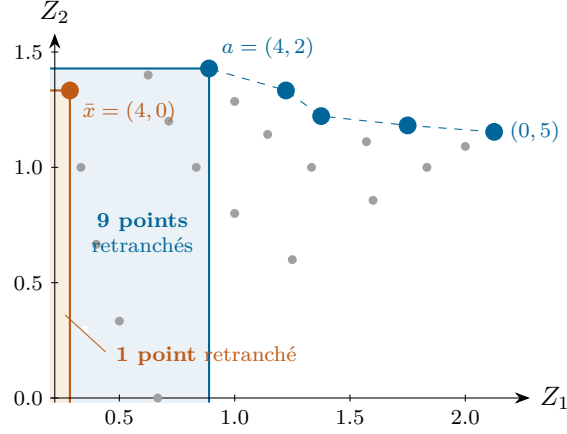
FIGURE 3 – Espace des critères de \mathcal{I}_2 : les 22 images, le front en bleu . La coupe de dominance en \bar{x} = (4, 0) retranche le rectangle orange – et ce rectangle ne contient qu' un seul point, \bar{x} lui-même : |\mathcal{R}| passe de 22 à 21. La coupe d' efficacité en a = (4, 2) retranche le rectangle bleu, qui en contient neuf : |\mathcal{R}_A| passe de 22 à 13. Même forme algébrique, même coût, neuf fois plus de matière. [sans mesure]
