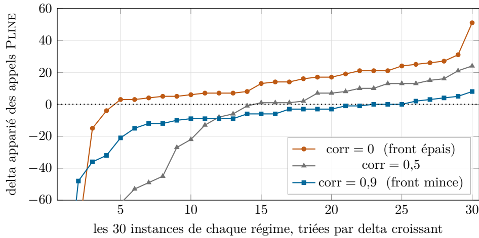
FIGURE 10 – Lecture appariée du lot de 90 instances : delta du nombre d’appels au solveur entier, instance par instance, trié dans chaque régime. Les valeurs hors cadre sont −205, −132, −129, −95, −83 et −81 – toutes des baisses . La figure dit ce qu’une médiane cache : à front mince la courbe est presque entièrement sous zéro, à front épais presque entièrement au-dessus, et le gain global tient à une queue courte de très fortes baisses plutôt qu’à un progrès réparti. C’est pourquoi la médiane appariée vaut +1 alors que le total baisse de 5,2 %. [Vo So Do]
