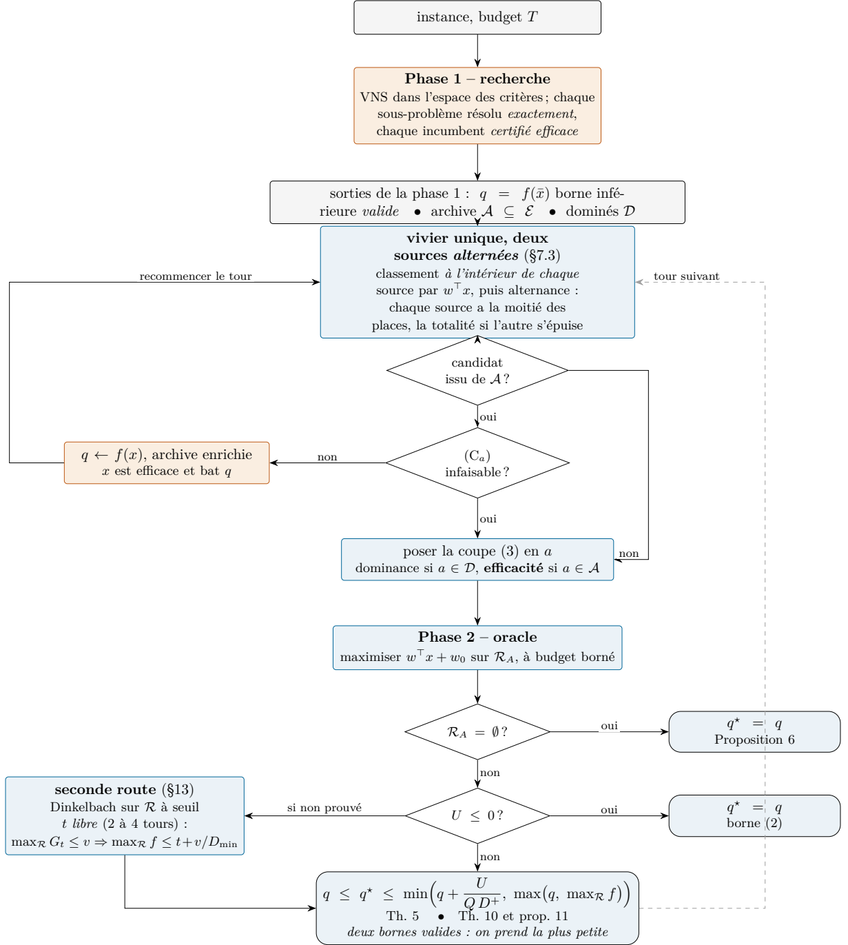
FIGURE 1 – Fonctionnement de l’algorithme, dans la configuration [V• S• D•] – celle que ce mémoire mesure partout. En orange ce qui existait, en bleu ce que la coupe d’efficacité ajoute. La flèche décisive est celle qui va de l’archive (sortie de la phase 1) au vivier de coupes de la phase 2 : c’est l’inversion du flux d’information qui fait l’hybridation. Deux éléments de ce schéma ont remplacé une version antérieure et la remplacent aussi dans le pseudo-code : l’ alternance du vivier, qui garantit des places à l’archive (§7.3), et la seconde route , qui évalue la même borne à un seuil libre (§13). L’état antérieur [V◦ S◦ D◦] est décrit à l’annexe A.
