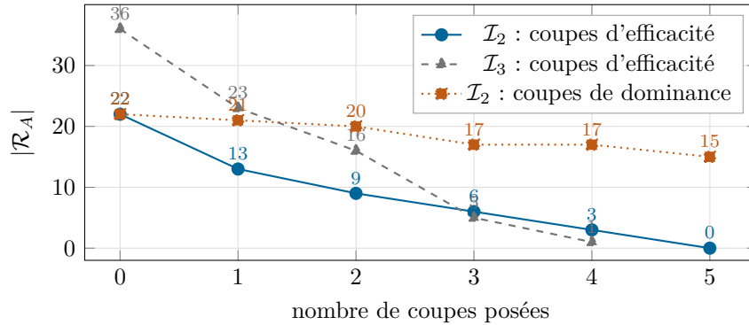
FIGURE 5 – Le relâché, coupe après coupe. Sur \mathcal{I}_2 la coupe d’efficacité le fait fondre de 22 points à zéro en cinq coupes – et un relâché vide est la preuve (proposition 6). La coupe de dominance, sur la même instance et pour le même nombre de coupes, descend de 22 à 15 : elle ne peut pas faire mieux, puisqu’elle préserve \mathcal{E} et se heurte donc au plancher |\mathcal{R}| \geq |\mathcal{E}| = 5 . Sur \mathcal{I}_3 la descente s’arrête à 1 : l’archive y est incomplète, il reste le point efficace non trouvé – et le théorème 5 conclut malgré tout, dès la deuxième coupe. [sans mesure]
