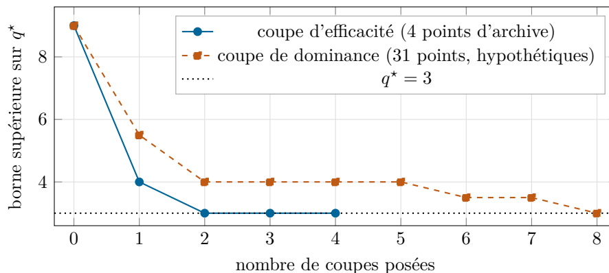
FIGURE 8 – \mathcal{I}_3 : même lecture qu’à la figure 6. L’écart de coût est ici d’un facteur 4 en nombre de coupes – donc en variables binaires ajoutées au programme entier. [sans mesure]
