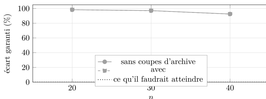
FIGURE 15 – Version antérieure , configuration [V◦ S◦ D◦], budget en temps. Les deux courbes sont confondues à 92–98 %. La légende d'origine expliquait ce plat ainsi : « la recherche produit assez de points dominés pour saturer le plafond avant que l'archive ne soit atteinte, de sorte qu'aucune coupe d'efficacité n'est posée ». Cette explication ne vaut que sous classement commun ; l'alternance la rend mécaniquement impossible. La figure 12 lui succède.
