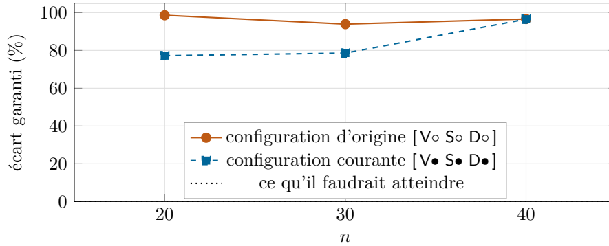
FIGURE 12 – La frontière honnête de la méthode, à front épais ( \text{corr} = 0 ), sous plafond déterministe de 300 appels entiers. Deux des trois points ont bougé de vingt et quinze points ; le troisième, n = 40 , n'a pas bougé du tout. La version antérieure de cette figure – deux courbes confondues à 92–98 % – et le diagnostic qui l'accompagnait sont à l'annexe A. [V◦ S◦ D◦] contre [V• S• D•]
