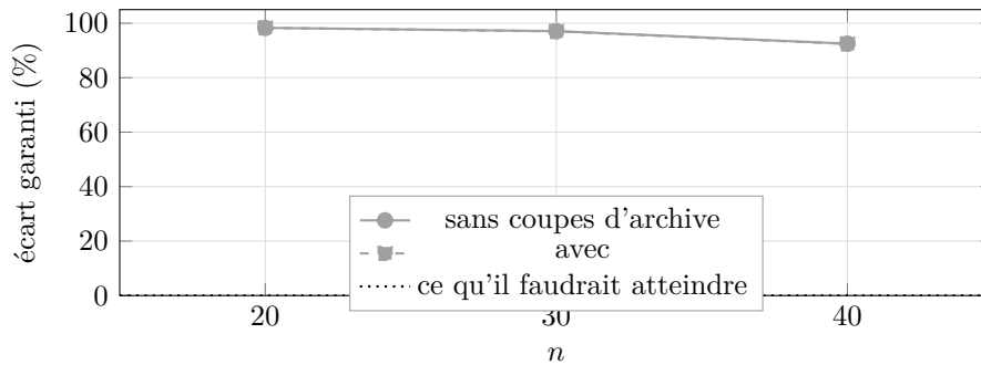
FIGURE 15 – Versión antérieure , configuration [V \circ S \circ D \circ] , budget en temps. Les deux courbes sont confondues à 92–98 %. La légende d'origine expliquait ce plat ainsi : « la recherche produit assez de points dominés pour saturer le plafond avant que l'archive ne soit atteinte, de sorte qu'aucune coupe d'efficacité n'est posée ». Cette explication ne vaut que sous classement commun ; l'alternance la rend mécaniquement impossible. La figure 12 lui succède.
