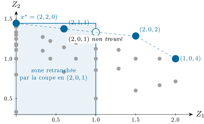
FIGURE 7 – \mathcal{I}_3 dans l'espace des critères (qui reste plan puisque p = 2 , même à n = 3 ). Le point efficace (2, 0, 1) , en cercle vide, n'est pas dans l'archive. La zone bleue est ce que retranche la coupe d'efficacité en (2, 0, 1) ... qu'on ne peut pas poser. C'est pourquoi \mathcal{R}_A ne se vide pas ici : il finit exactement sur ce point.
