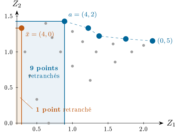
FIGURE 3 – Espace des critères de \mathcal{I}_2 : les 22 images, le front en bleu . La coupe de dominance en \bar{x} = (4,0) retranche le rectangle orange – et ce rectangle ne contient qu’un seul point, \bar{x} lui-même : |\mathcal{R}| passe de 22 à 21. La coupe d’ efficacité en a = (4,2) retranche le rectangle bleu, qui en contient neuf : |\mathcal{R}_A| passe de 22 à 13. Même forme algébrique, même coût, neuf fois plus de matière.
