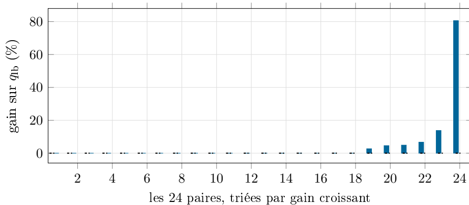
FIGURE 11 – Diversification par coupes d'efficacité, à budget d'appels identique. Aucune barre ne descend sous zéro : sur les 24 paires, la valeur rendue n'est jamais dégradée. Dix-huit paires sont exactement nulles, six montent, de +2,7 à +80,6 %. C'est cette asymétrie – rien à perdre, parfois beaucoup à gagner – qui justifie le mécanisme, bien plus que sa moyenne.
