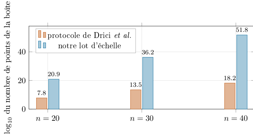
FIGURE 14 – Pourquoi « n = 40 » ne désigne pas le même problème. Des contraintes tirées sur [1, 30] avec un second membre sur [50, 100] bornent les variables par 2 ou 3 ; les nôtres le sont par 19 en médiane. À la même valeur de n , trente-quatre ordres de grandeur séparent les deux boîtes. Prouver 80/80 sur le protocole de gauche ne dit rien du régime de droite – et c’est ce dernier qui nous résiste.
