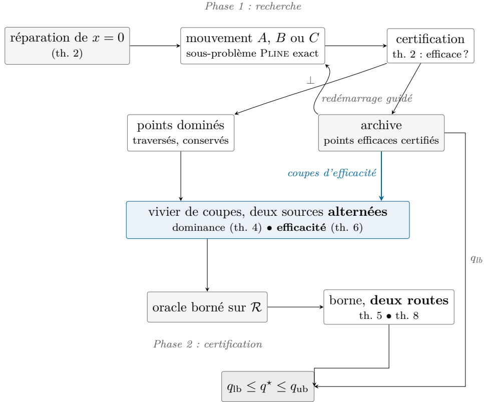
FIGURE 5 – Architecture, dans la configuration [V \bullet S \bullet D \bullet] – celle que ce travail mesure partout. La phase de recherche ne produit que des points certifiés efficaces, d’où une borne inférieure jamais optimiste. Elle alimente la phase 2 par deux canaux : les points dominés qu’elle traverse, sur lesquels le théorème 4 autorise une coupe, et l’ archive , sur laquelle le théorème 6 en autorise une autre – c’est la flèche bleue, et c’est la contribution. Les deux sources alternent dans le vivier plutôt que d’y être classées ensemble, faute de quoi l’archive est affamée (§15) ; et la borne finale est le minimum de deux routes valides, l’une à seuil fixé sur l’incumbent, l’autre à seuil libre (§15). Le budget non consommé par la recherche est reversé à la certification.
