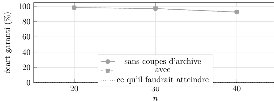
FIGURE 15 – Version antérieure , configuration [V\circ S\circ D\circ] , budget en temps. Les deux courbes sont confondues à 92–98 %. La légende d'origine expliquait ce plat ainsi : « la recherche produit assez de points dominés pour saturer le plafond avant que l'archive ne soit atteinte, de sorte qu'aucune coupe d'efficacité n'est posée ». Cette explication ne vaut que sous classement commun ; l'alternance la rend mécaniquement impossible. La figure 12 lui succède.
