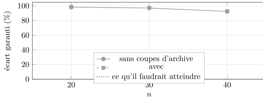
FIGURE 15 – Versión antérieure , configuration [V\circ S\circ D\circ] , budget en temps. Les deux courbes sont confondues à 92–98 %. La légende d'origine expliquait ce plat ainsi : « la recherche produit assez de points dominés pour saturer le plafond avant que l'archive ne soit atteinte, de sorte qu'aucune coupe d'efficacité n'est posée ». Cette explication ne vaut que sous classement commun ; l'alternance la rend mécaniquement impossible. La figure 12 lui succède.
