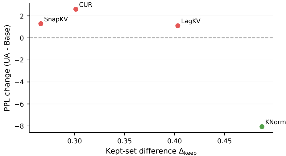
(d) Selection Difference
