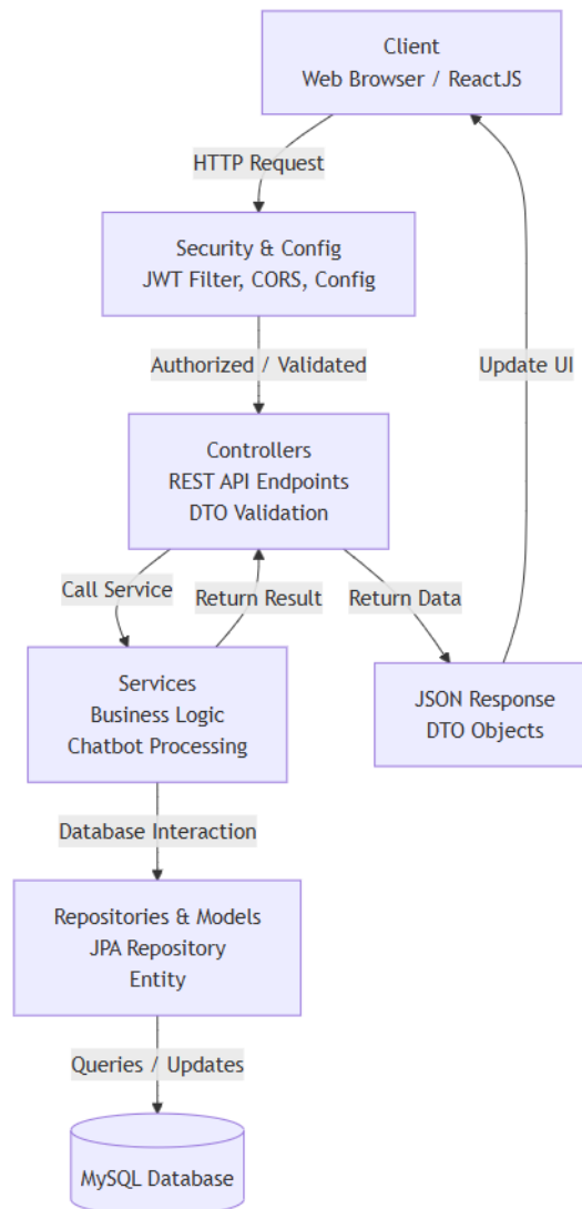
Hình 3. 8 Sơ đồ mô tả luồng xử lý của chatbot AI
