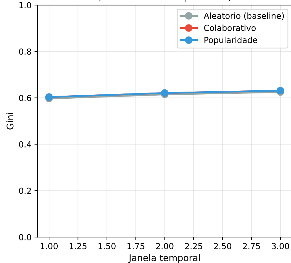
Índice de Gini (Concentração de Popularidade)
