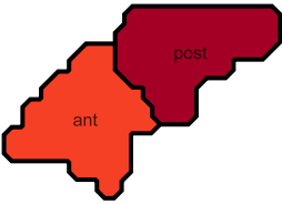
PreCG
