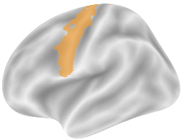
Cortical ROIs
