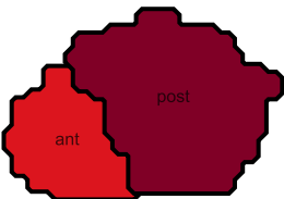
Putamen
