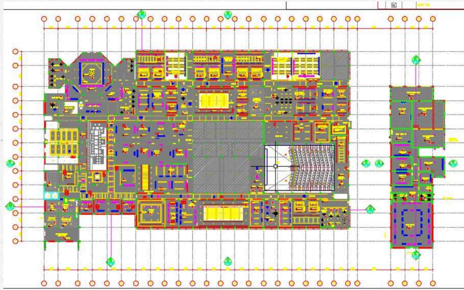
CEILING-PLAN
