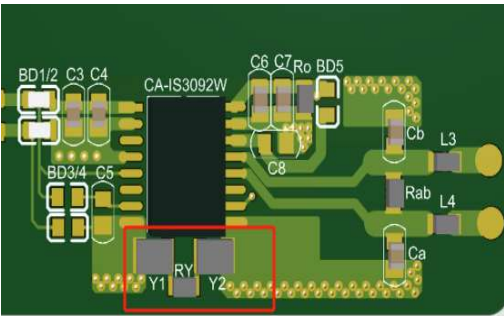
PCB 3D 图
