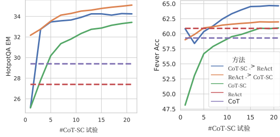
图2: PaLM-540B在不同CoT-SC样本数量下的提示结果。
