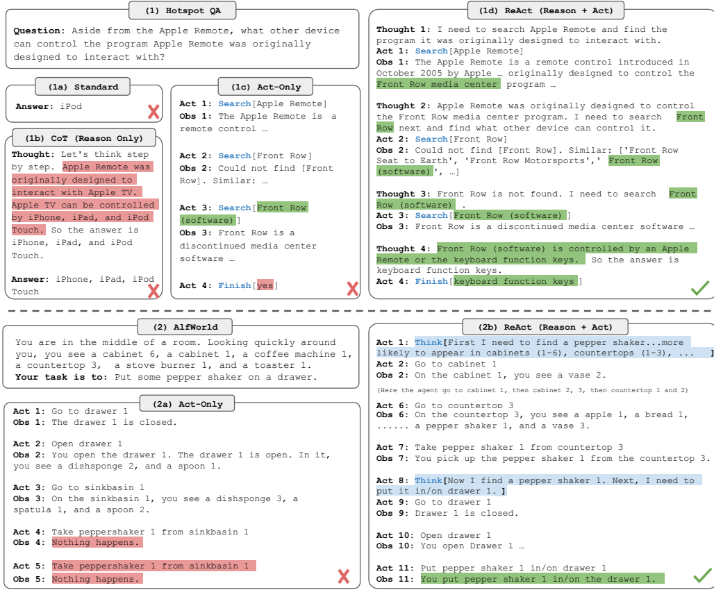
图1: (1) 四种提示方法的比较, (a) 标准方法, (b) 连锁思维 (CoT, 纯推理), (c) 仅行动 (Act-only), (d) ReAct (Reason+Act), 用于解决HotspotQA (Yang等, 2018) 问题。 (2) (a) 仅行动提示与(b) ReAct提示在解决AlfWorld (Shridhar等, 2020b) 游戏中的比较。在两个领域中, 我们省略了提示中的上下文示例, 仅显示模型生成的任务解决轨迹 (行动、思考) 和环境 (观察)。
