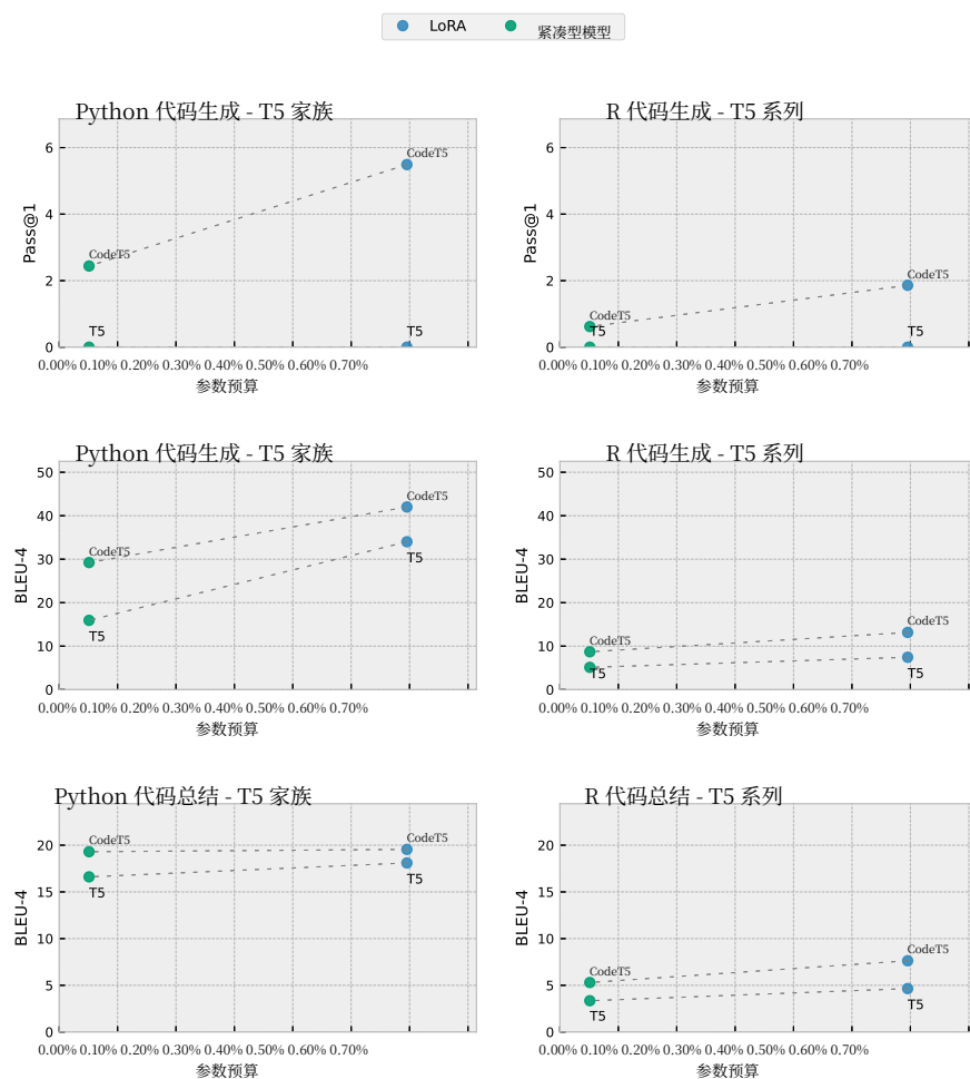
图 3 使用 T5 系列模型进行 Python 和 R 代码生成及摘要任务中，Compacter 和 LoRA 的性能与可训练参数预算关系。BLEU-4 表示性能。参数预算是指训练参数占总参数数量的百分比。
