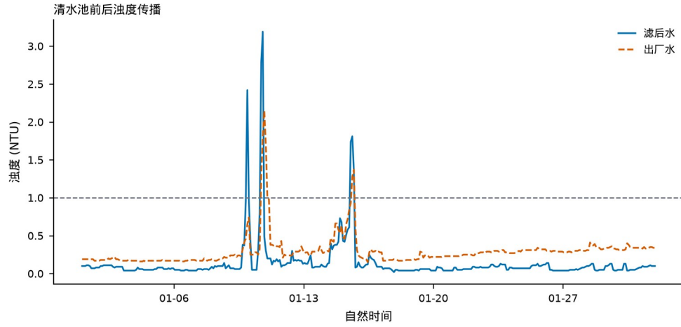
2026 年 1 月清水池前后浊度传播
