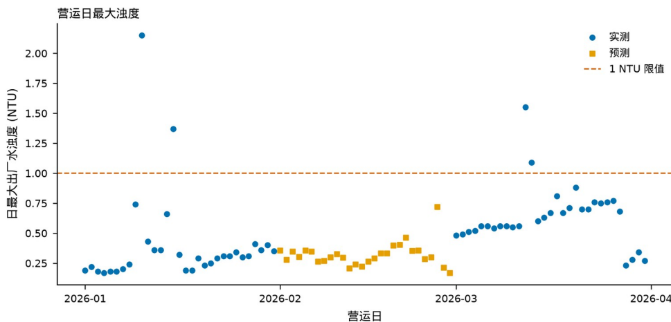
90 个营运日的最大出厂水浊度
