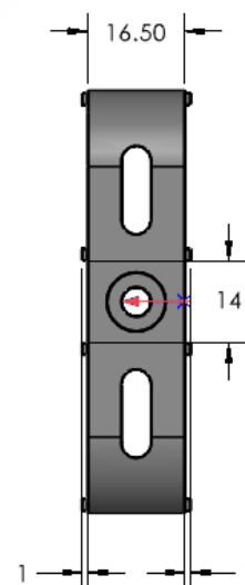
DETAIL D (28X) SCALE 5 : 1
