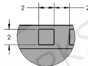
DETAIL D (28X) SCALE 5 : 1
