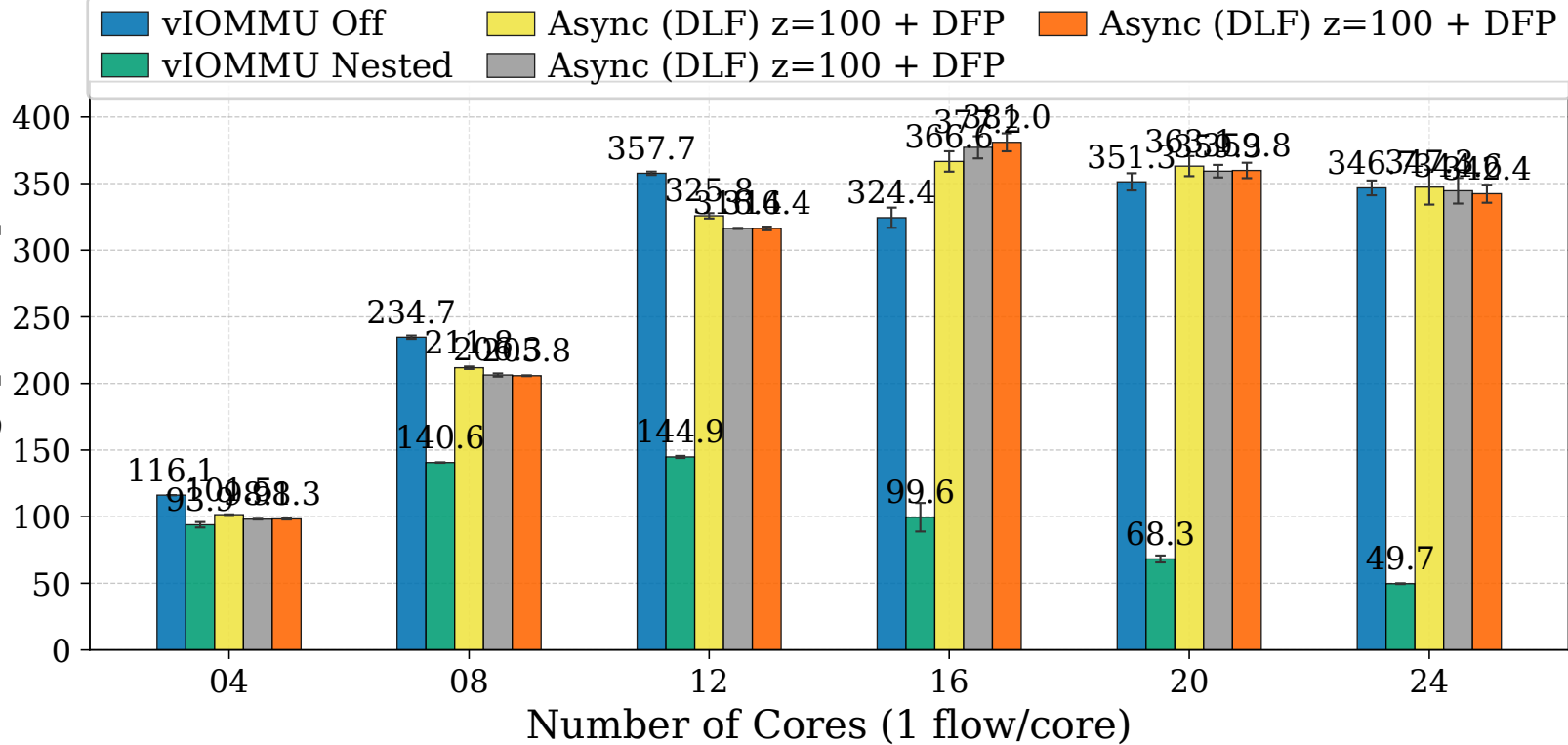
Throughput (Gbps)
