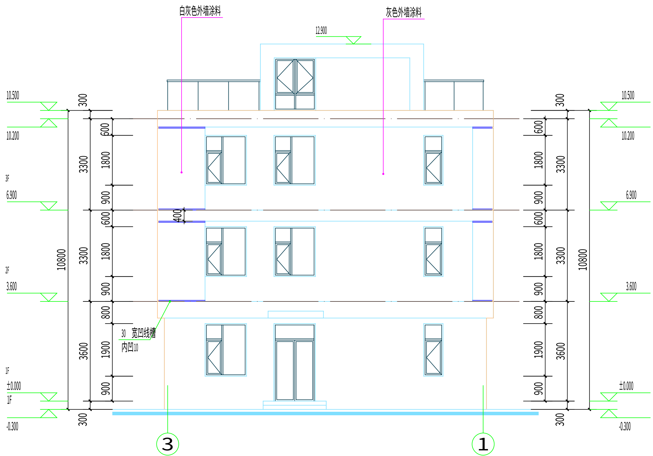
北立面图 1:100
