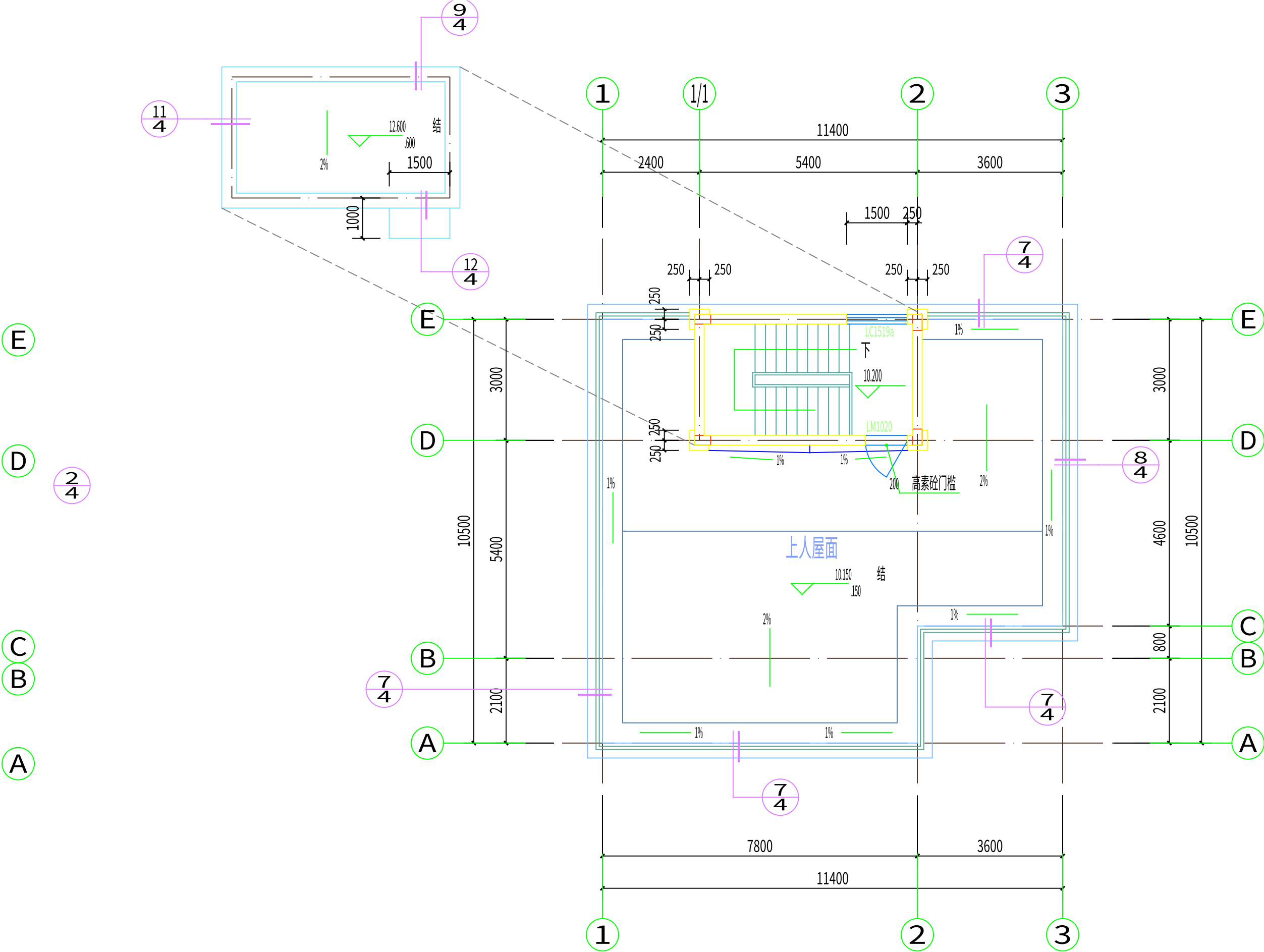
屋顶平面图
