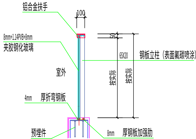
玻璃栏板1-1剖面图 1:25
