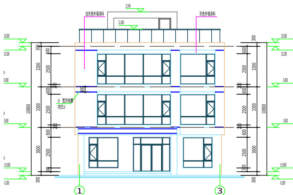
南立面图 1:100
