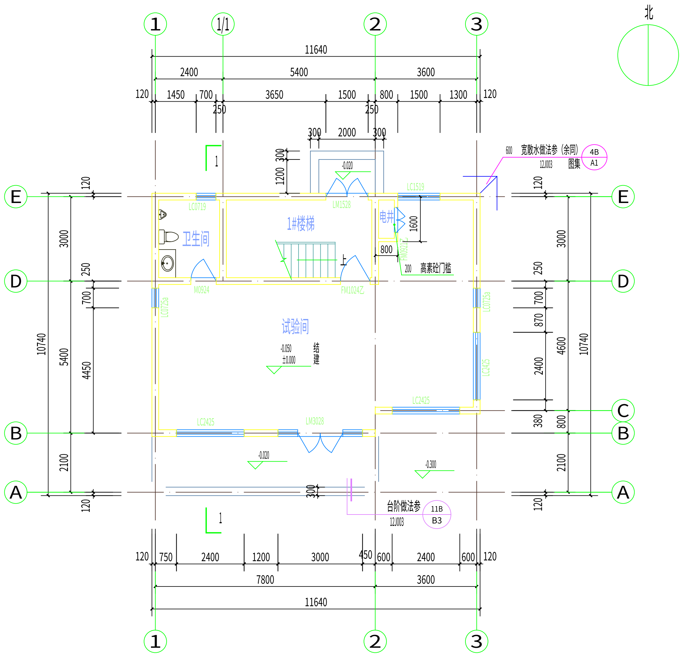
一层平面图 1:100
