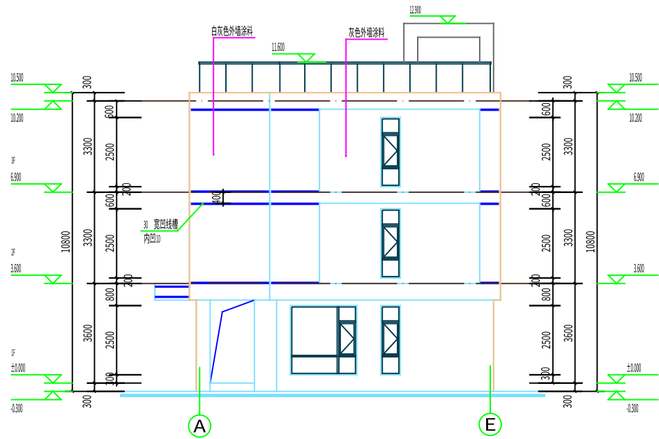
东立面图 1:100
