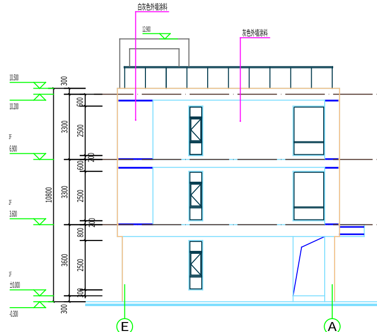
西立面图 1:100
