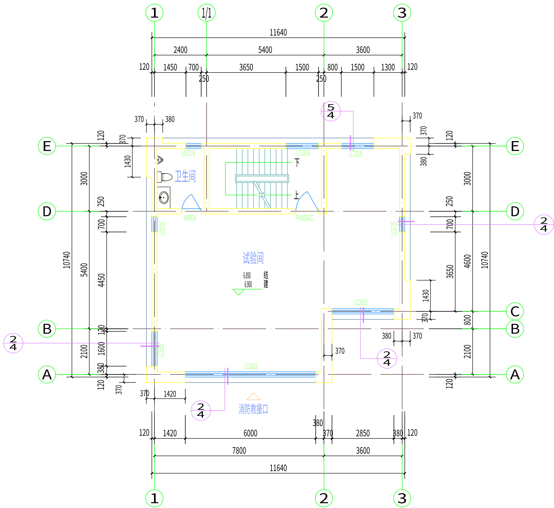
三层平面图 1:100
