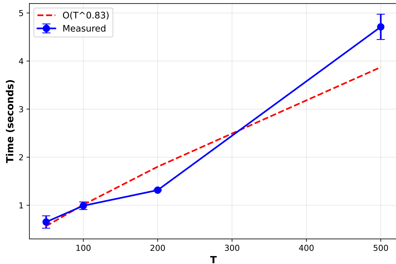
Runtime vs T (Linear Scale)
