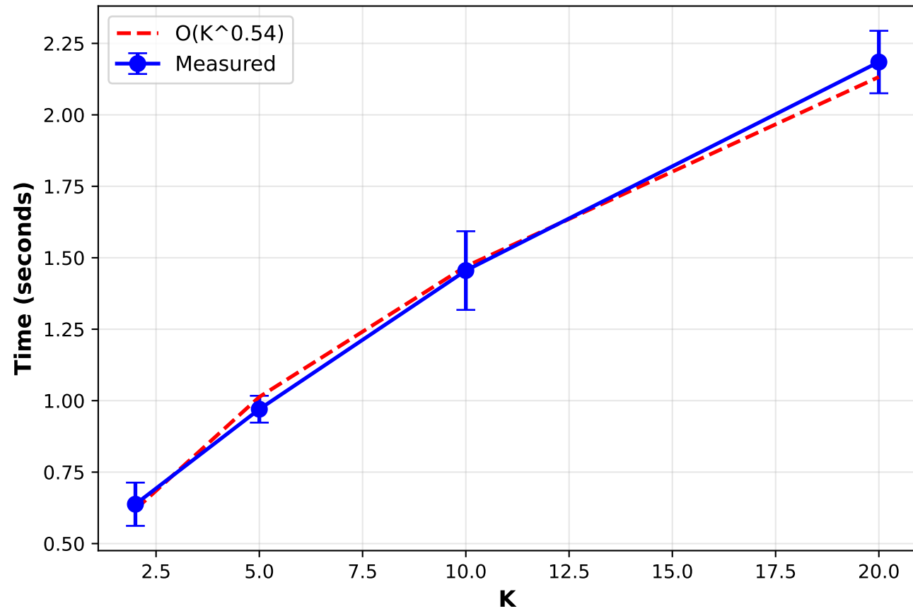
Runtime vs K (Linear Scale)
