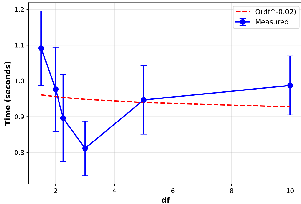
Runtime vs df (Linear Scale)
