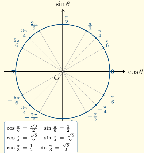
Cercle trigonométrique
