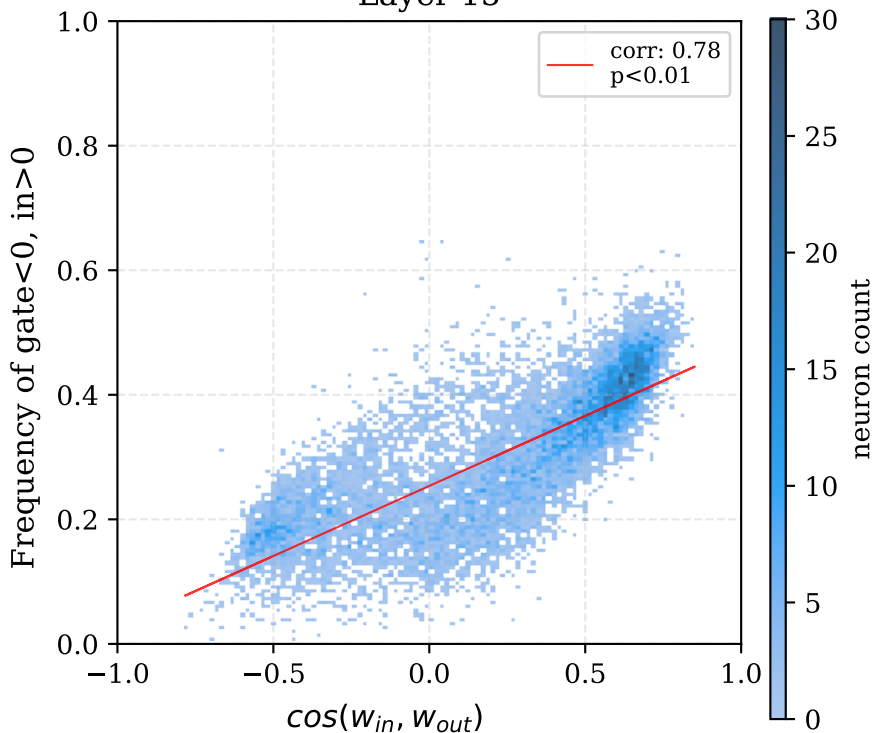
Layer 15
