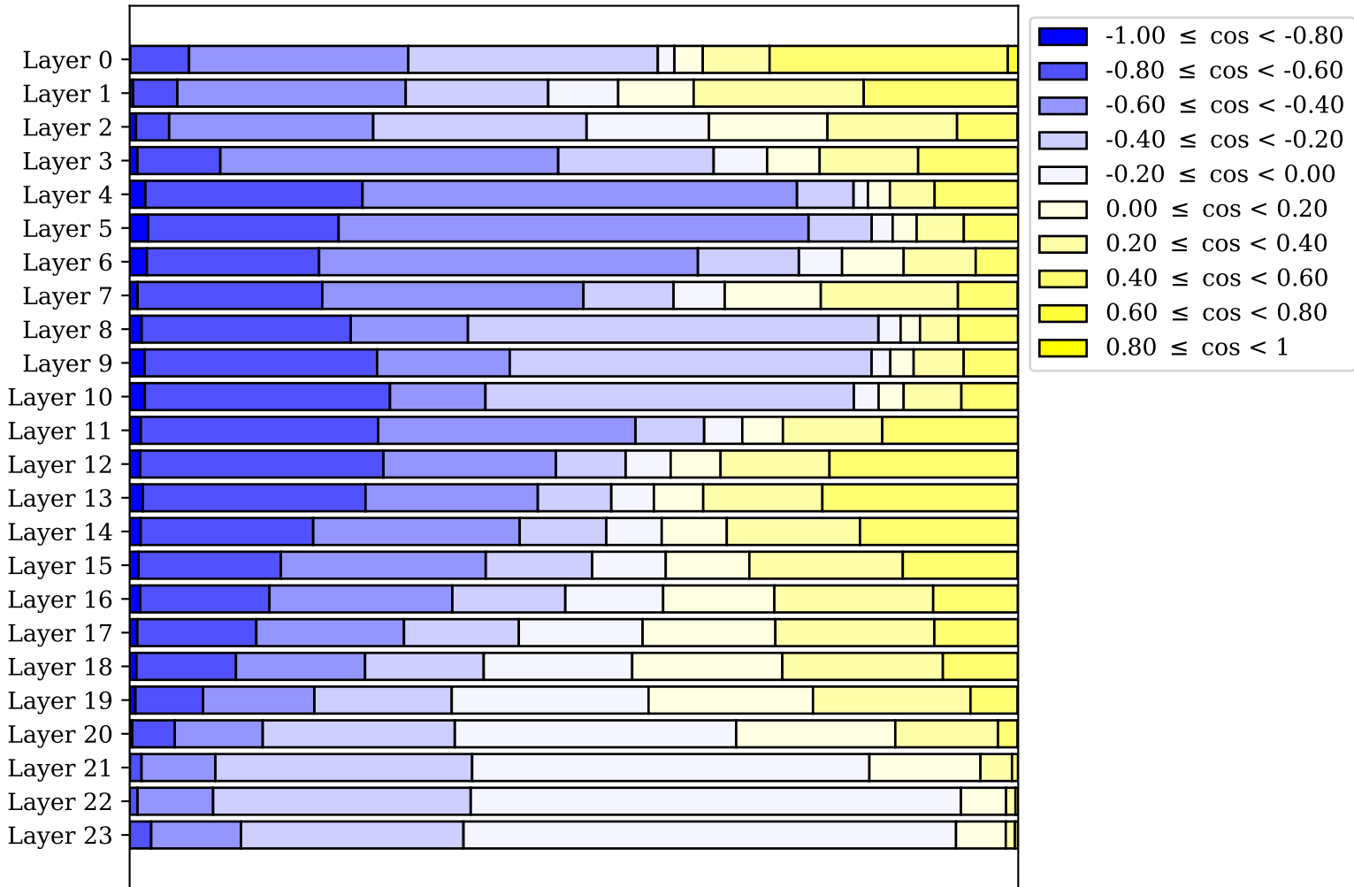
bloom-1b1
